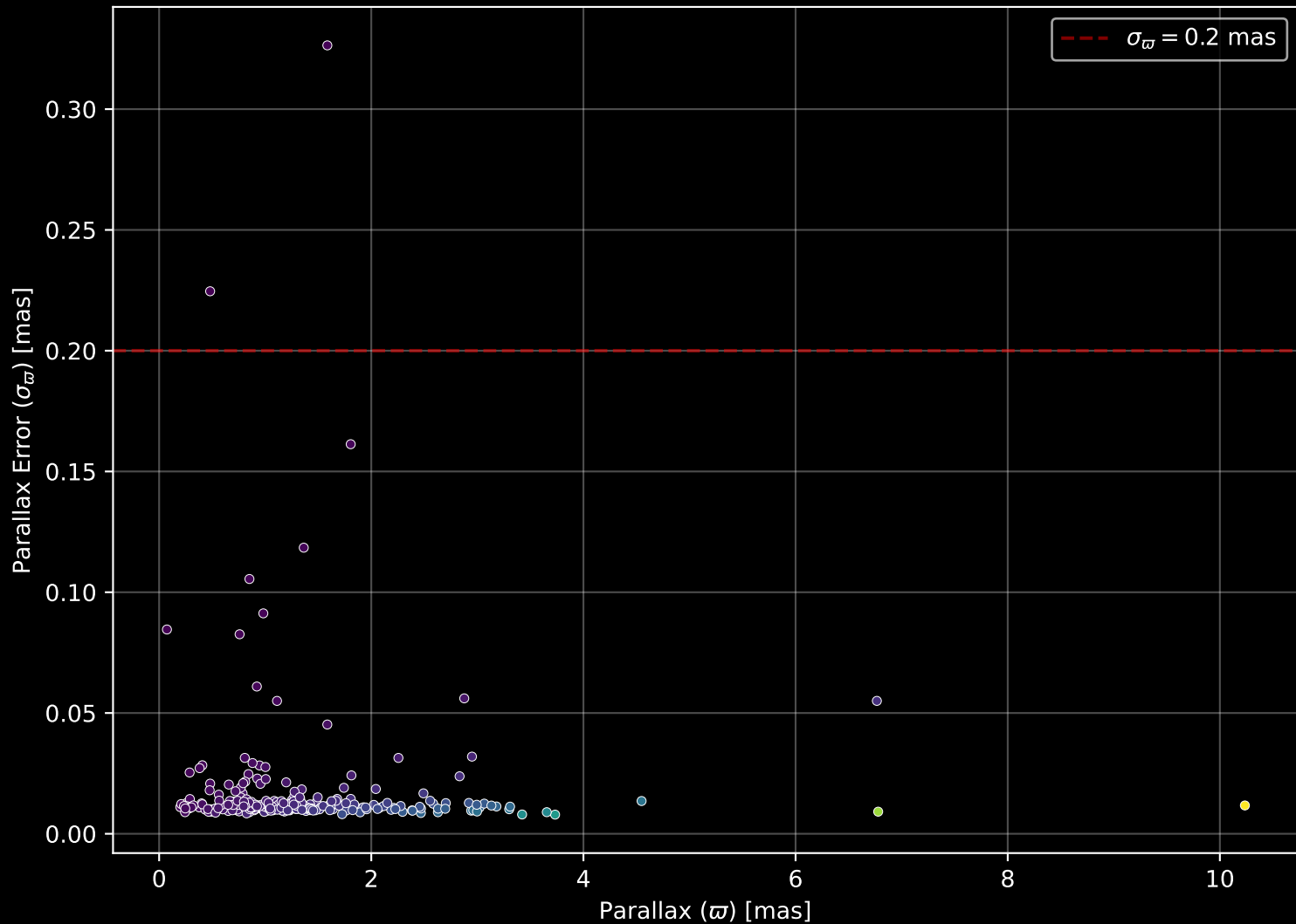
GALAH DR4 Field: [2439] Parallax Quality (n= 271)
