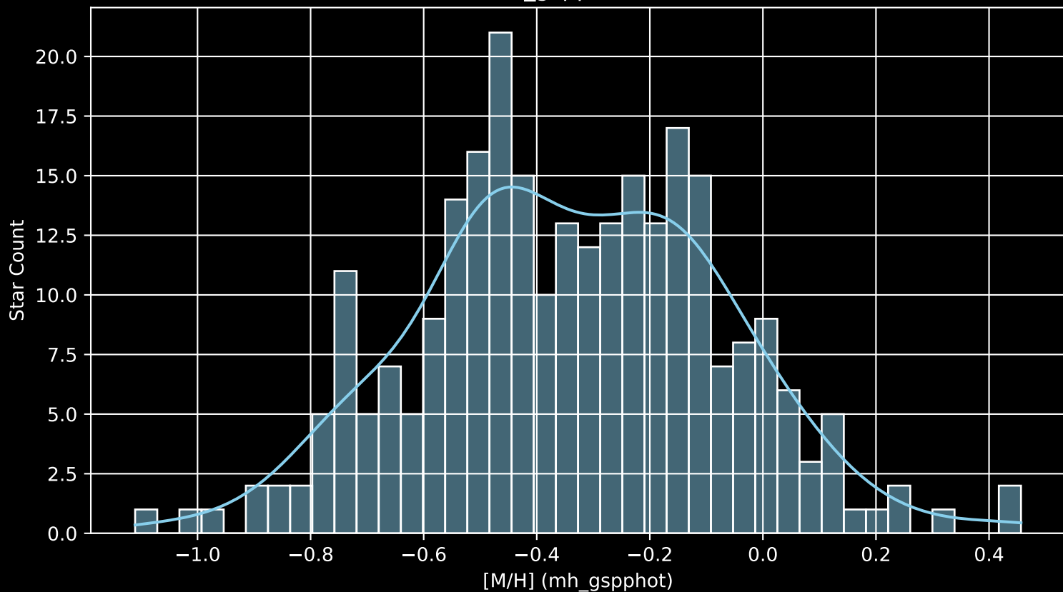
GALAH DR4 Field: [2439] [M/H] (mh_gspphot) (n= 270)
