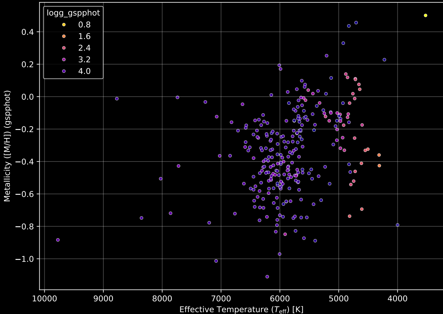
GALAH DR4 Field: [2439] Stellar Population Parameters (n= 271)
