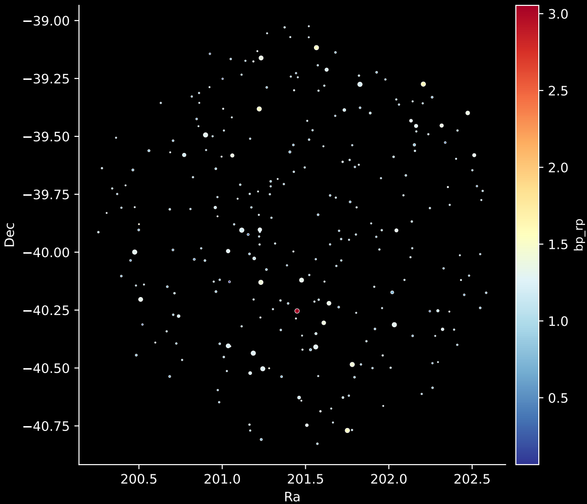
GALAH DR4 Field: [2439] Stars: 271
